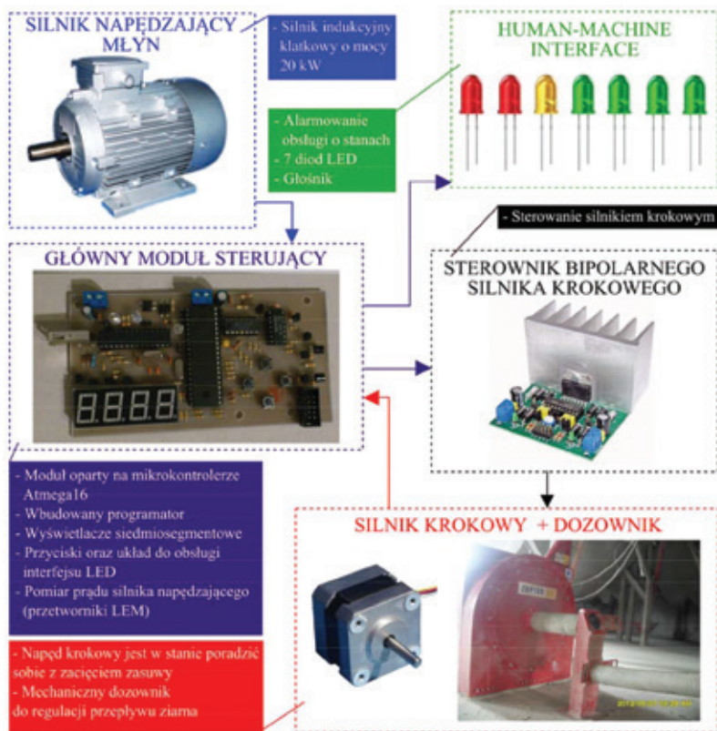
Rys. 1. Schemat ideowy układu sterownika dozownika
