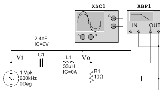
Rys. 11. Szeregowy obwód RLC prądu zmiennego
