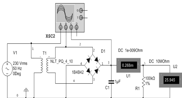
Rys. 13. Prostownik dwupółkowny z mostkiem Graetza z filtrem
