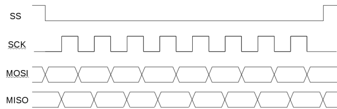
Rys. 1. Przebiegi na magistrali SPI między mikrokontrolerem a układem CPLD
