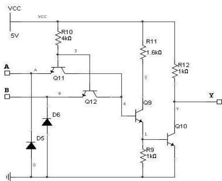
Rys. 8. Struktura wewnętrzna podobudowu NAND_OC
